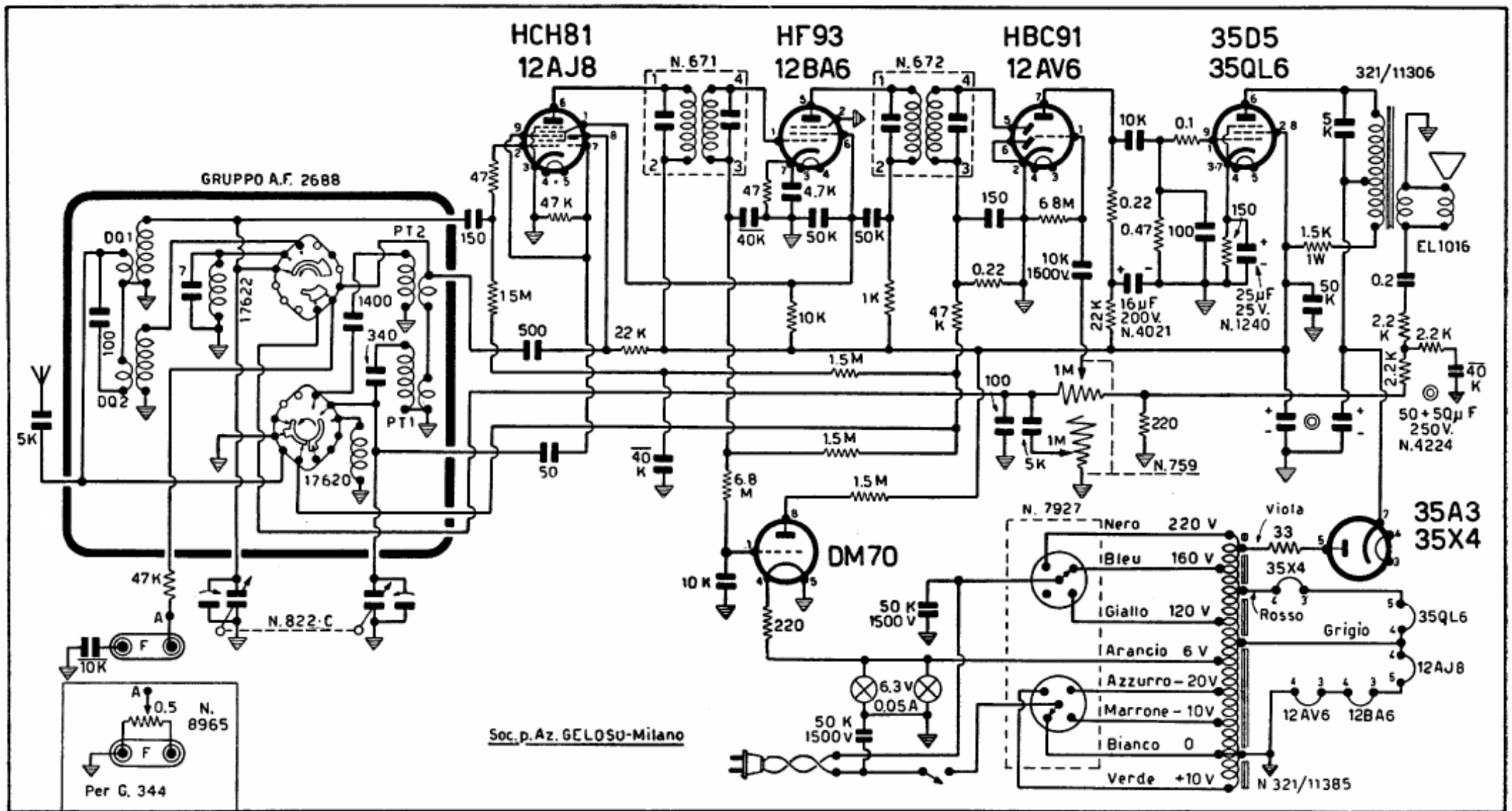
Schema elettrico del ricevitore G 334-A
